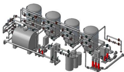
Установка по водоподготовке
